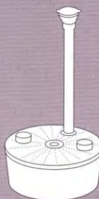
Mona Tank 10 Vandindhold: 10 l Diameter 38,5 cm, Højde 10 cm Påfyldningsrør 46 cm
